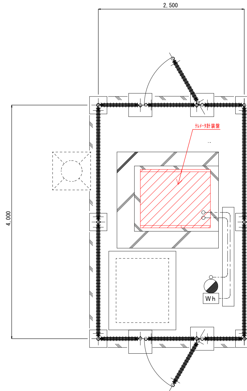
平面図 S=1/20
