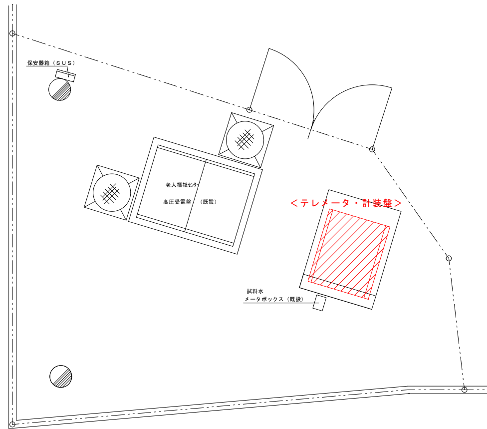
第1低区末端圧検出所 平面図 S=1/30
