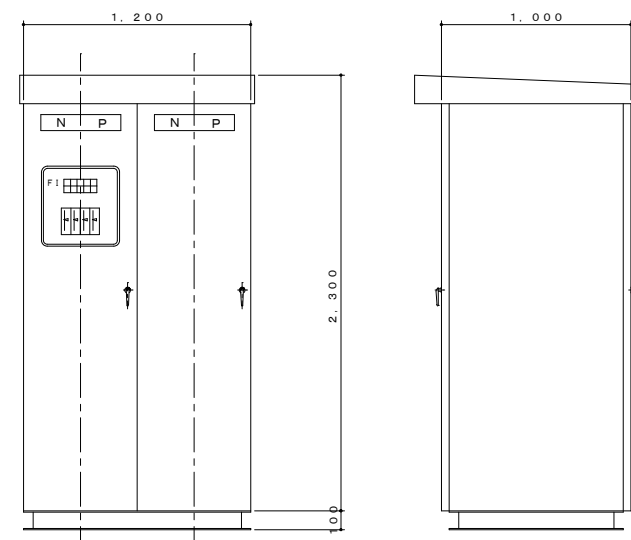
テレメータ・計装盤
