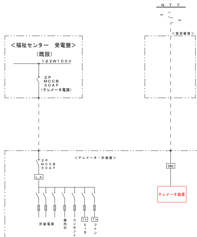
単線結線図
