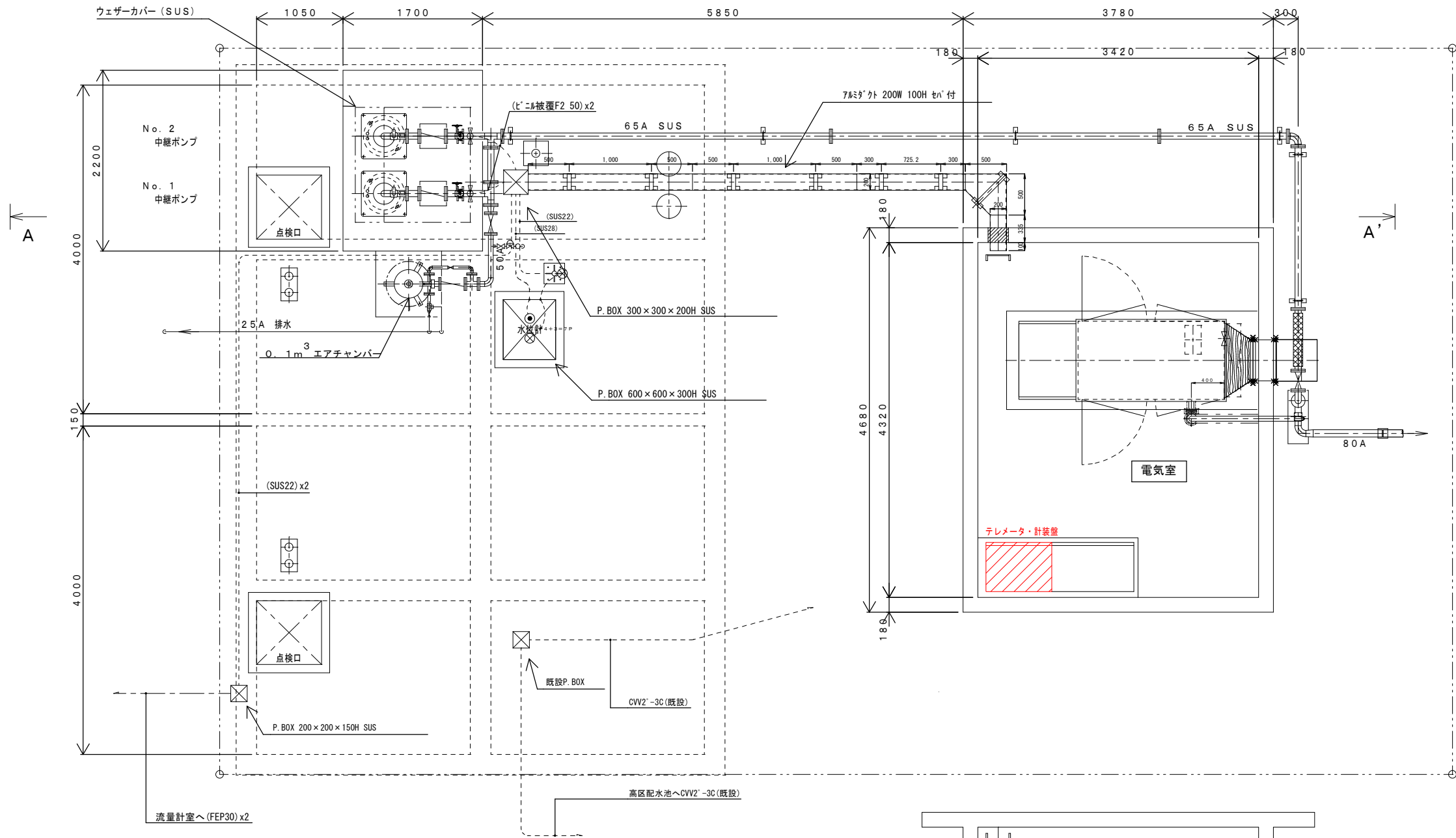
平面図 S=1/30
