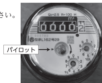
< 水道メーターの一例 >
