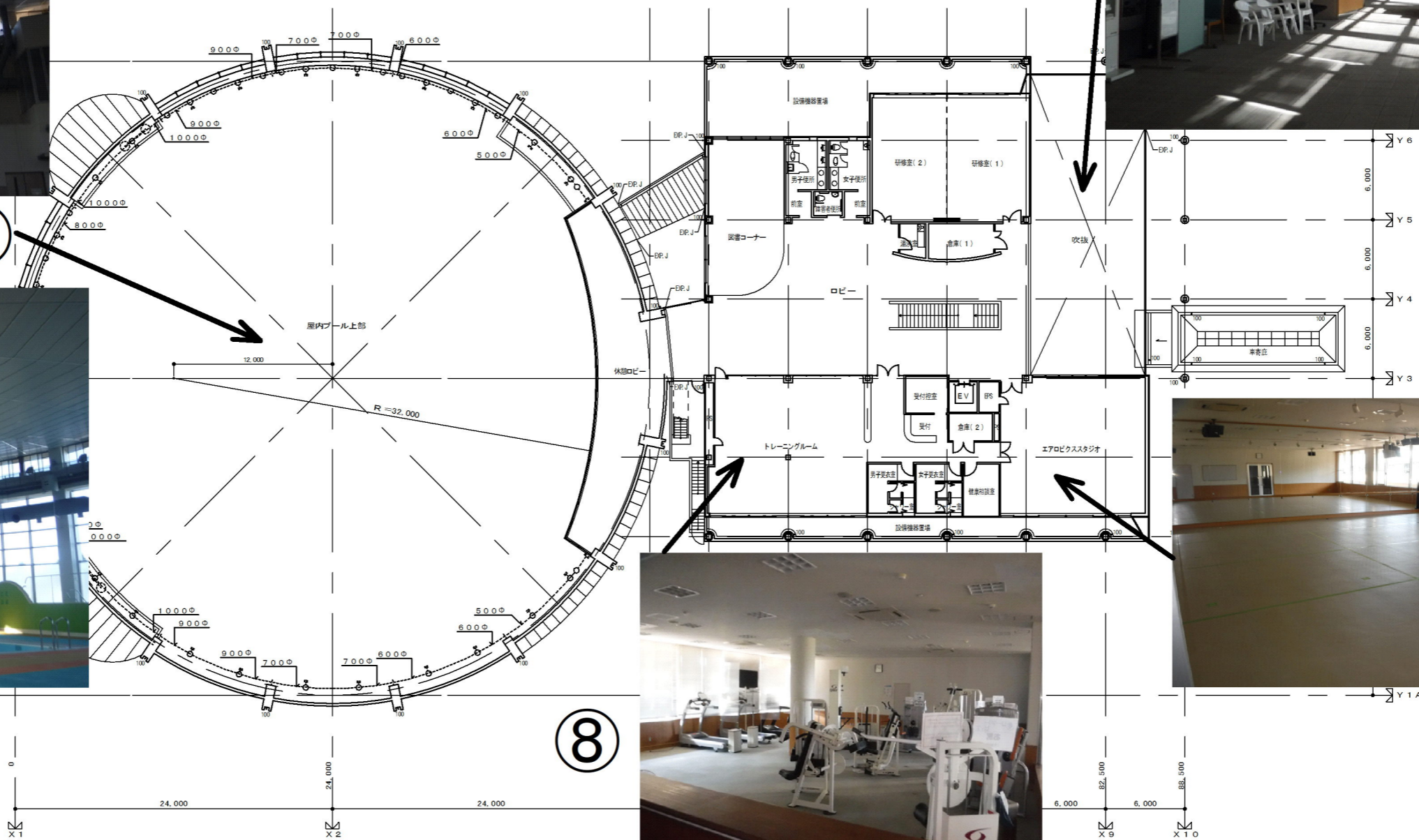
2階平面図 1/200
